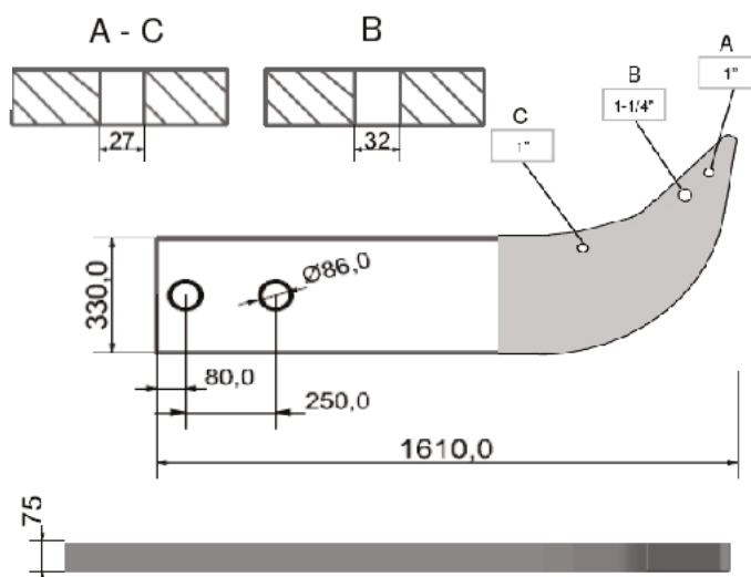
Detalle Taladro Pasadores
