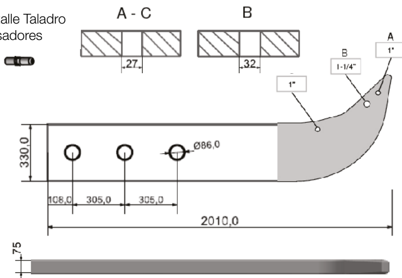
Detalle Taladro Pasadores
